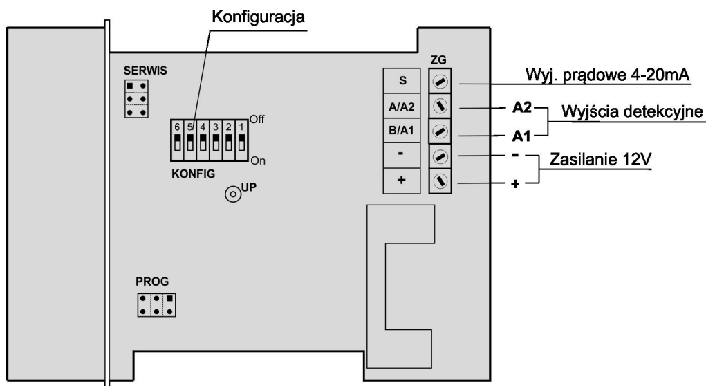
Rys.3. Listwa zaciskowa Detektora Gazów Palnych "EXpert G"
