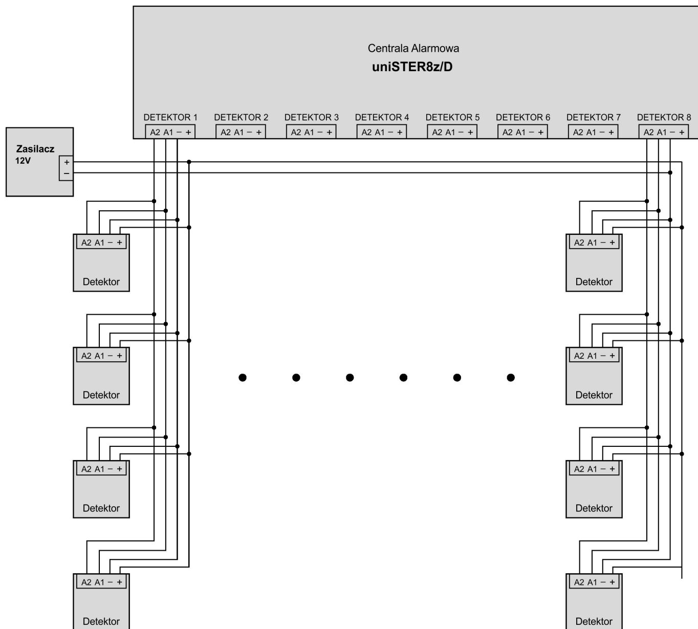
Rys.7. Przykładowe połączenie strefowe detektorów „EXpert G” z centralą „uniSTER8z/D” (8 stref - po 4 detektory)
