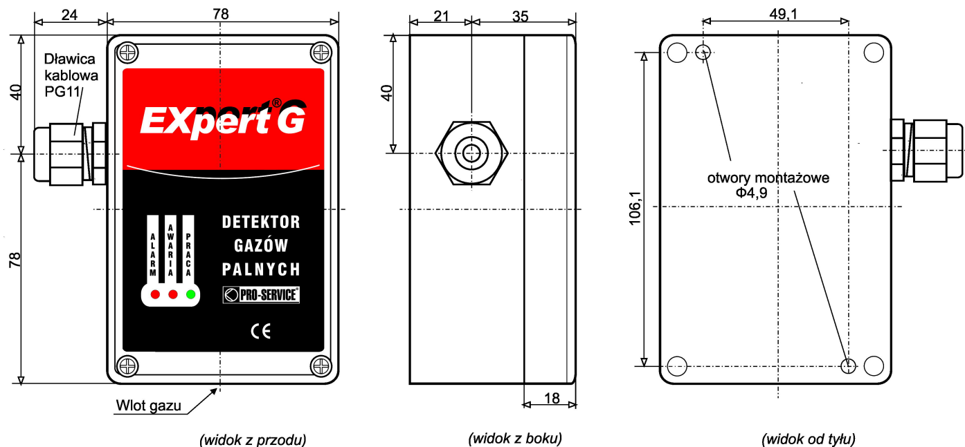
Rys.5. Wymiary - detektory „Expert G /K” (z sensorem katalitycznym), „Expert G /E” (z sensorem elektrochemicznym), „Expert G /IR” (z sensorem infradrowym)
