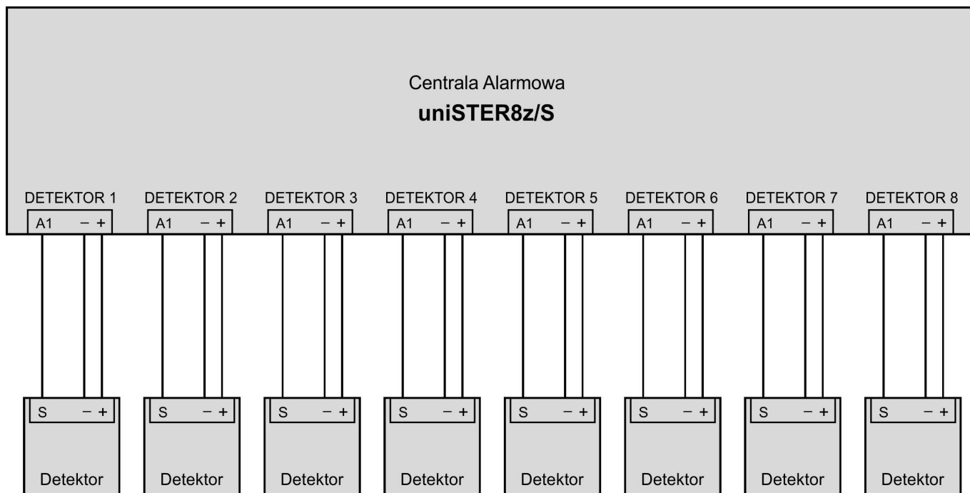
Rys.8. Połączenie Detektorów Gazów Palnych „EXpert G” z centralką uniSTER8z/S, przy wykorzystaniu wejść prądowych 4_20mA.
