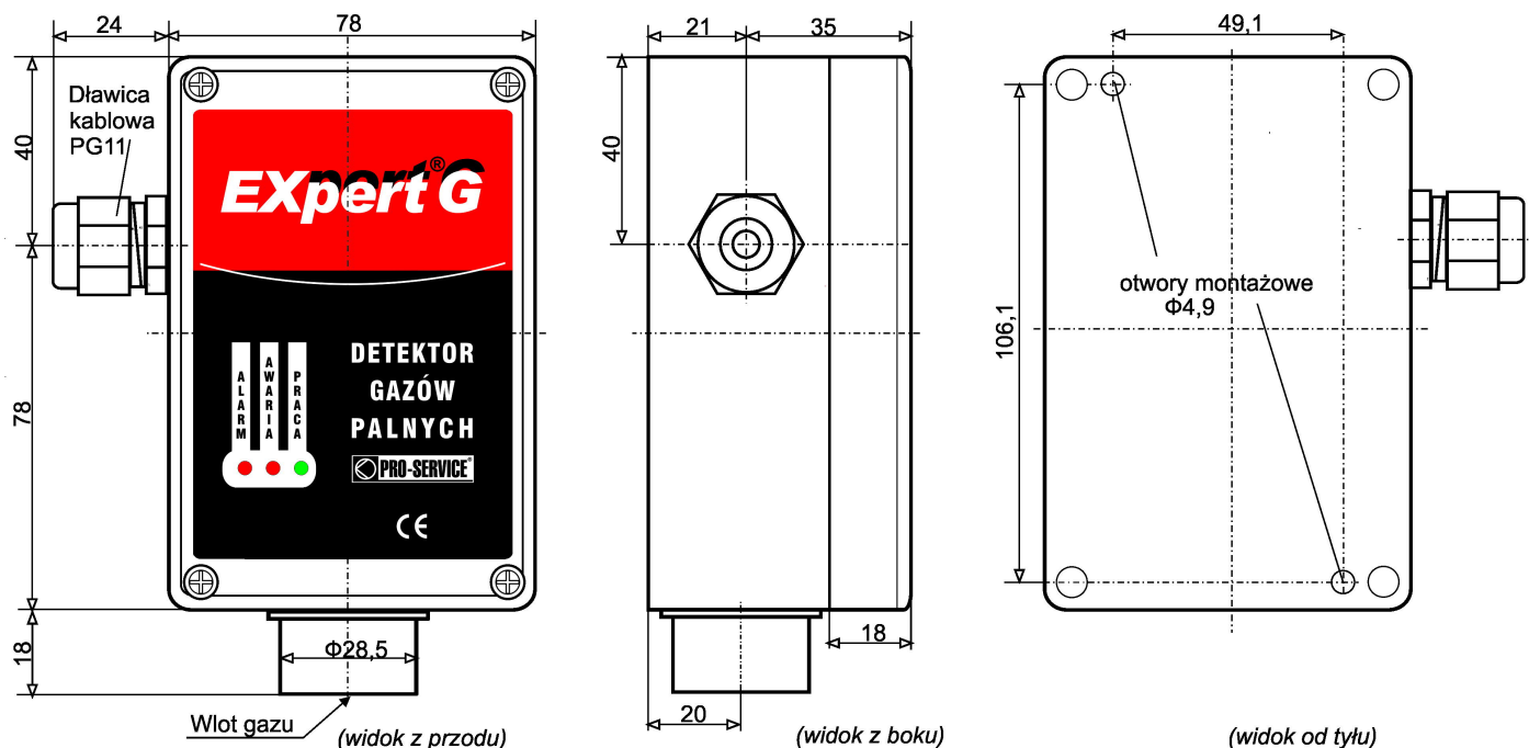
Rys.4. Wymiary Detektora Gazów Palnych „Expert G /PP” ( z sensorem półprzewodnikowym)
