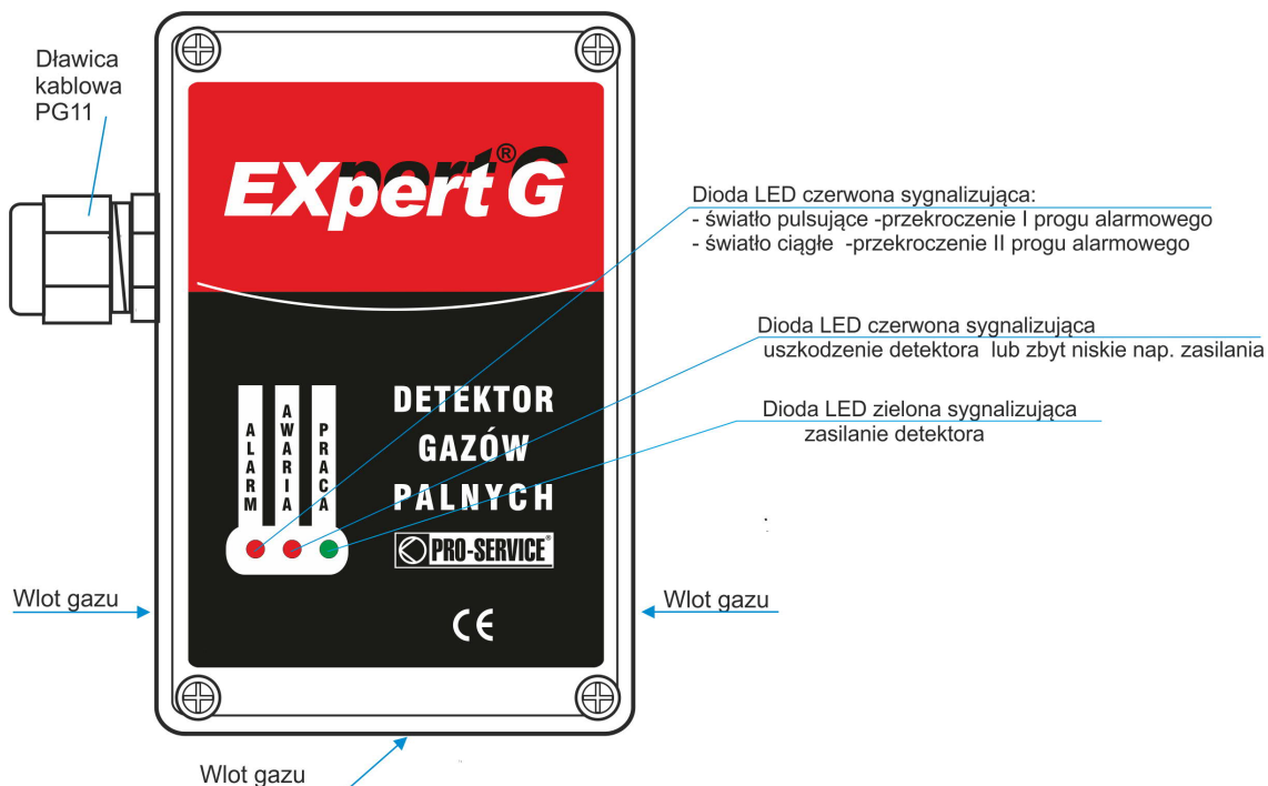
Rys.2. Widok - detektory „Expert G /K” (z sensorem katalitycznym), „Expert G /E” (z sensorem elektrochemicznym), „Expert G /IR” (z sensorem infradowym)
