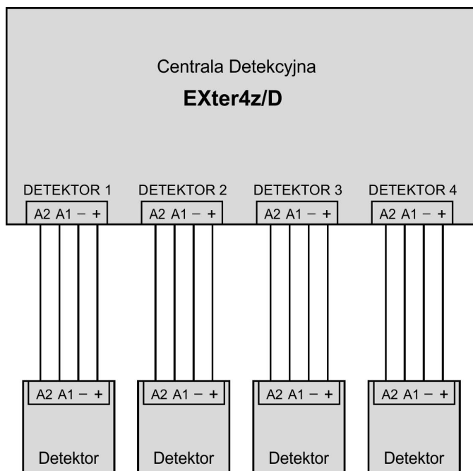
Rys.6. Podłączenie Detektora Gazów Palnych „EXpert G” do centralki Exter4z
