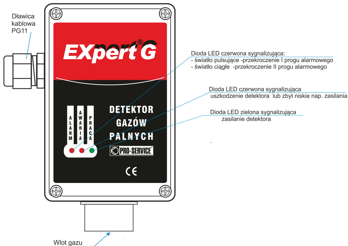
Rys.1. Widok - detektor „Expert G /PP” ( z sensorem półprzewodnikowym)
