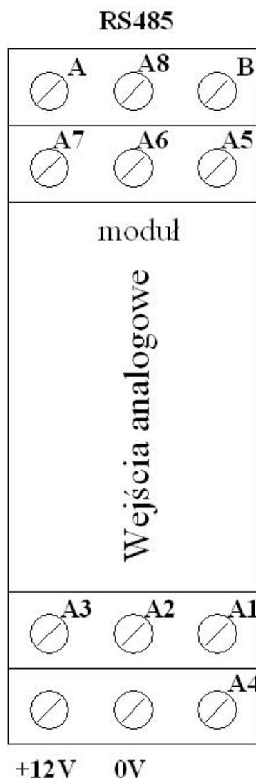
Rys. 15. – Listwy zaciskowe modułu wejść analogowych 4-20mA centrali modularPAG®.
