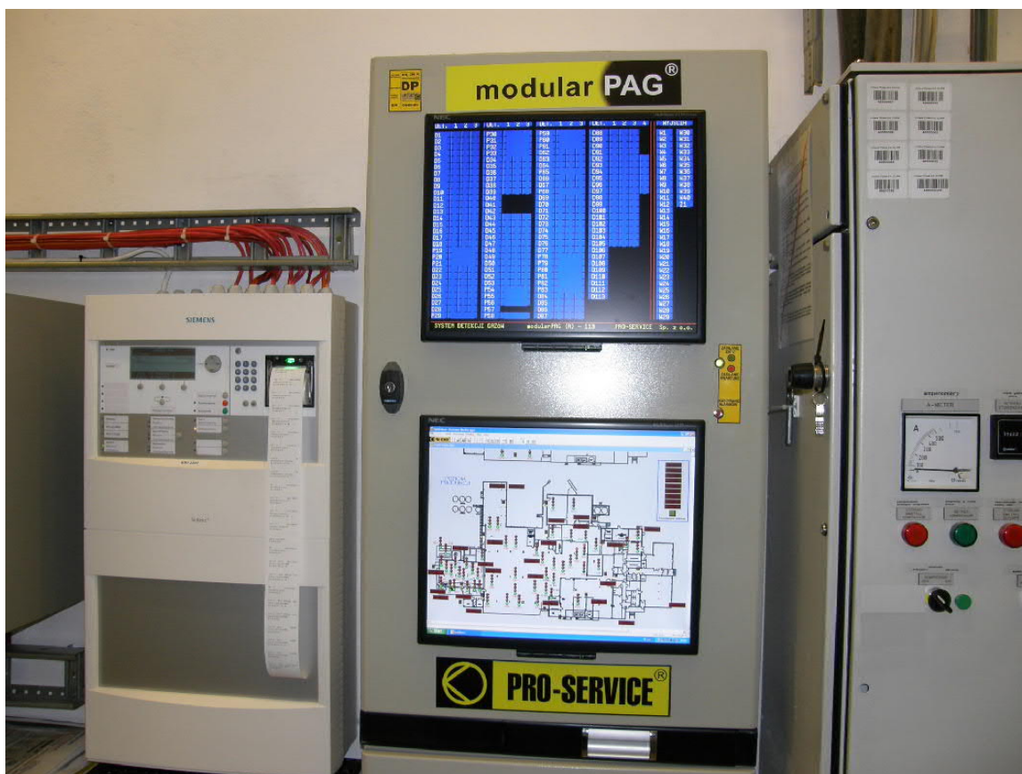
Rys. 21. – Centrala modularPAG® wraz z systemem wizualizacji PAG®view.
