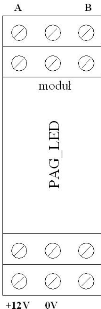
Rys. 16. – Listwy zaciskowe modułu sygnalizacji LED centrali modularPAG®.
