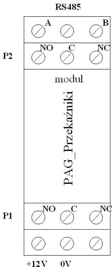
Rys. 14. – Listwy zaciskowe modułu dodatkowych wyjść przełącznikowych centrali modularPAG®.
