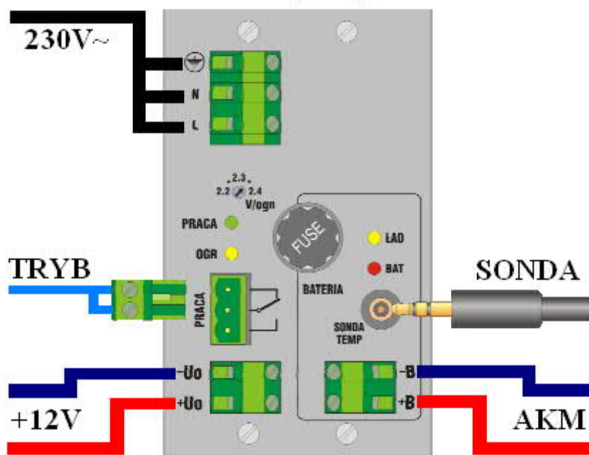
Rys. 12. – Płyta czołowa modułu zasilacza centrali modularPAG®.
