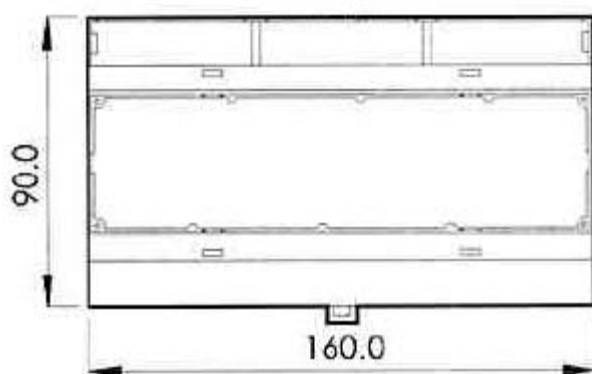
Rys. 8. – Wymiary modułu sterującego centrali modularPAG ® .
