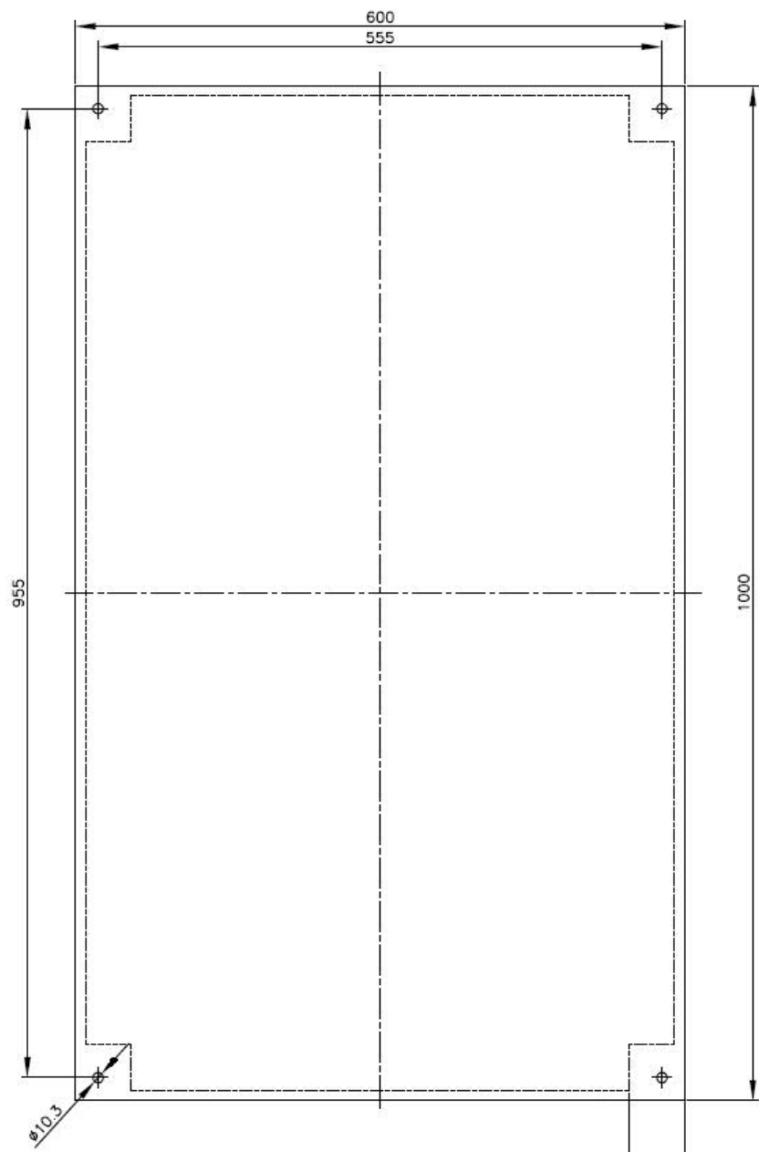
Rys. 6. – Wymiary szafy instalacyjnej 600mm x 1000mm x 250mm stosowanej jako obudowa dużej wielkości centrali modularPAG®.
