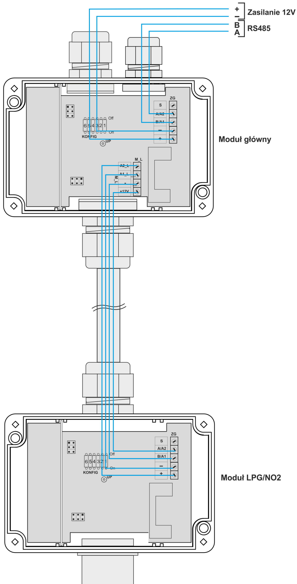
Rys.2. Tmaster CO/LPG/NO2 G/EPE/RS485 – listwy zaciskowe, połączenie modułu głównego i modułu LPG/NO2
